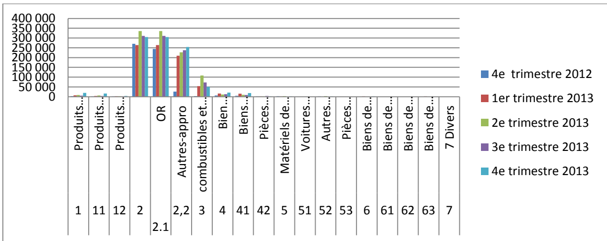
Graphique 4 : Exportation de l'OR et des autres approvisionnements industriels de la période
